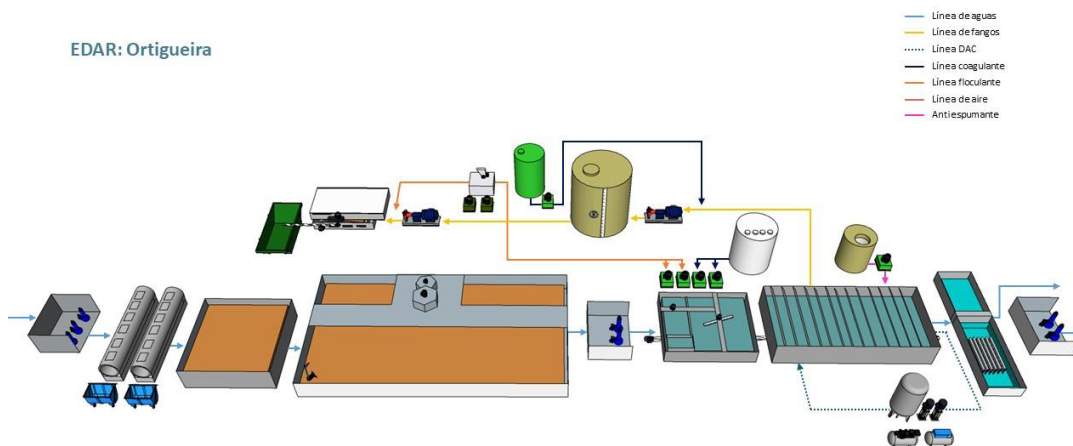
Diagrama de fluxo do proceso de depuración da EDAR de Ortigueira
