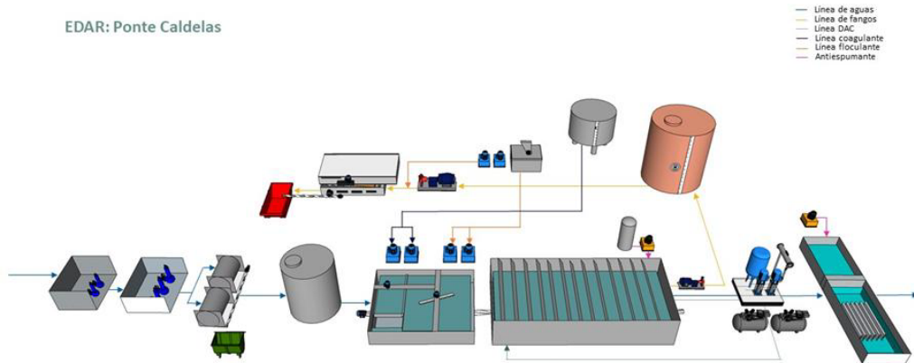
Figura 4. Diagrama de proceso da EDAR
